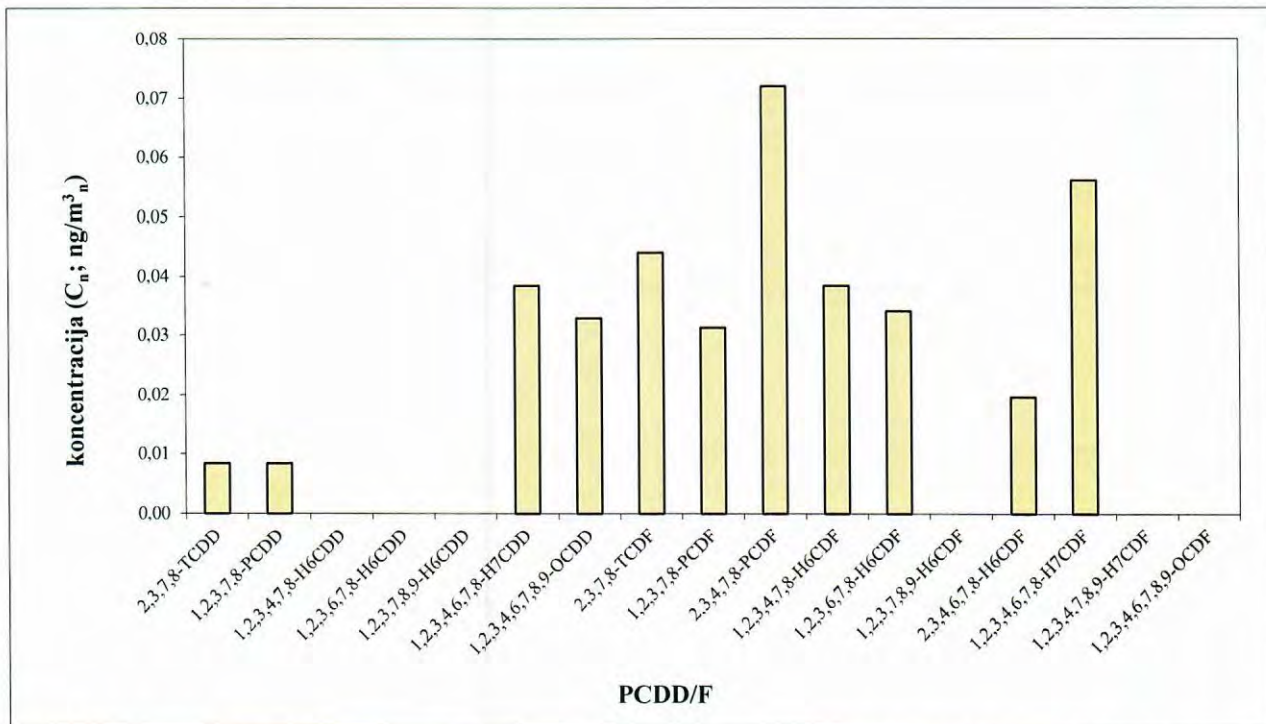
SLIKA 1: Porazdelitev masnih koncentracij posameznih 2,3,7,8-izomer polikloriranih dibenzodioxinov (PCDD) in polikloriranih dibenzofuranov (PCDF)
